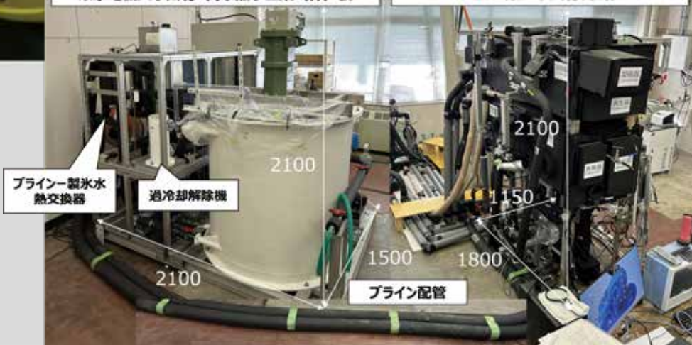
3kW氷点下冷熱用吸収冷凍機 八戸工業大学所有、製作
